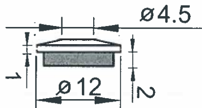
Рис.2 Уплотнительная шайба для резьбовых шпилек X-BT и X-BT-MF
