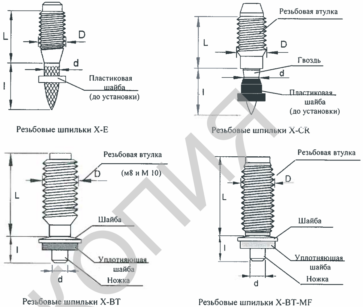
Рис. 1 Общий вид резьбовых шпилек
