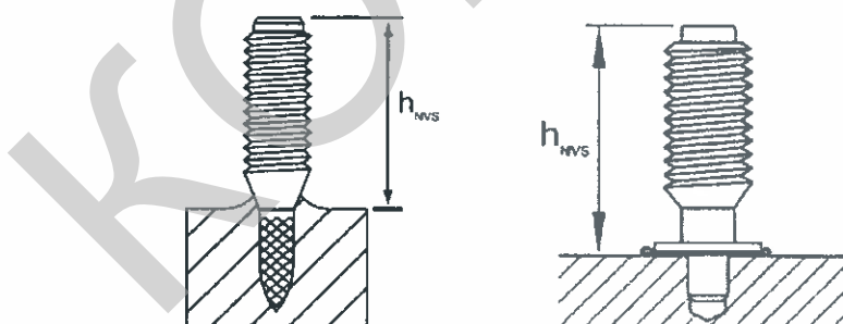
Рис.4 Величина выступа h NVS для резьбовых шпилек
