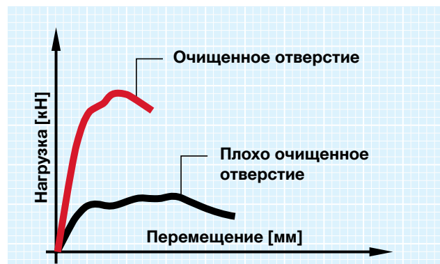
Выраженное влияние качества очистки отверстия
