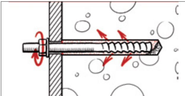
HIT-Z с химическим анкером Hilti HIT-HY 200-A
